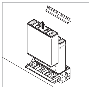
Staffa di montaggio a parete
