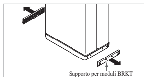
Supporto per moduli BRKT
